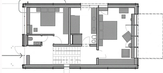
1. STĀVA PLĀNS
