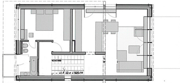
2. STĀVA PLĀNS
